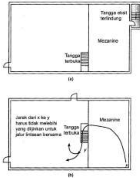
Contoh 3.27 - Jumlah sarana jalan ke luar dari mezanine (sebagai tambahan penjelasan butir 3.12.1.1)
