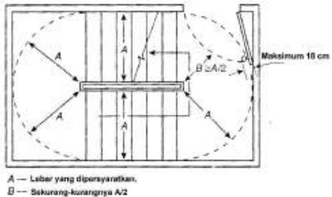
Contoh 3.11 - Minimum jarak antara tak terhalangi yang disyaratkan dengan pintu yang mengganggu pada bordes dalam bangunan gedung baru (sebagai penjelasan butir 3.7.1.4)
