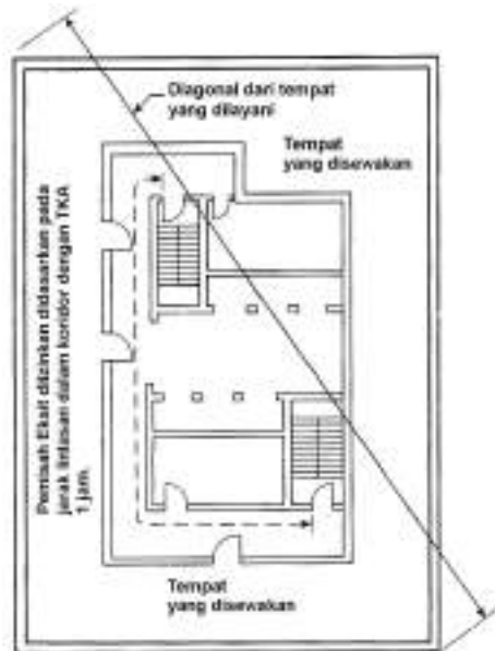
Gambar A.3.13.1.3.2.(d) - Pemisah eksit diukur sepanjang lintasan koridor.
