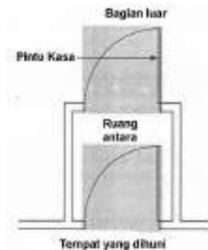
Contoh 3.13 - Susunan ruang antara ( vestibule ) yang menuju pintu kaca memenuhi butir 3.7.1.6
