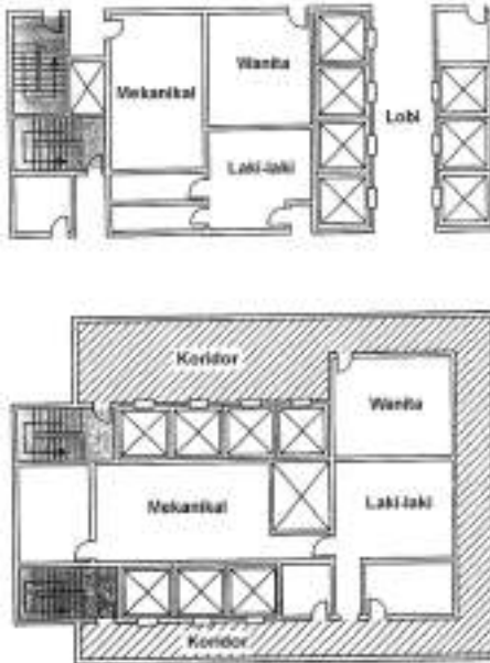
Contoh 3.32 - Akses ke eksit pada core bangunan gedung yang banyak penyewa. (sebagai penjelasan tambahan butir 3.13.1.3.2)
