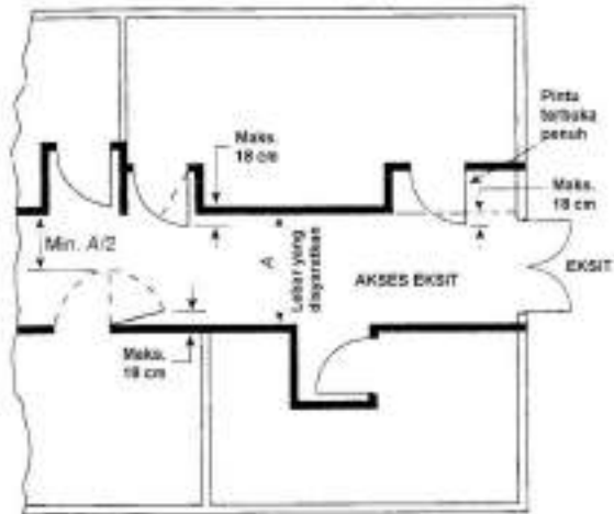
Contoh 3.10 - Pintu yang membuka ke dalam koridor. (sebagai penjelasan butir 3.7.1.4)
