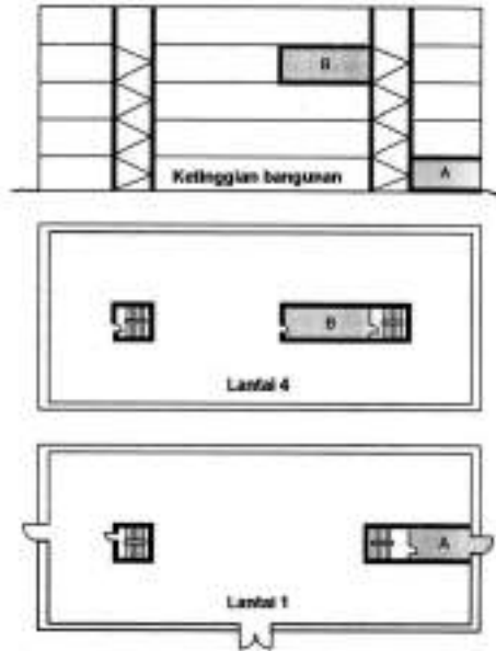
Contoh 3.20 – Jalan Terusan Eksit terlindung (A dan B) tahan api dan pintu tahan api (sebagai penjelasan tambahan butir 3.9.3)
