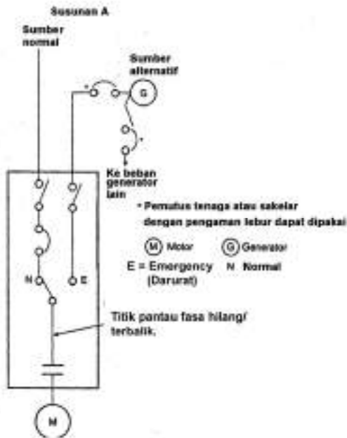
Gambar 6.1.4.2.(a) - Susunan A
