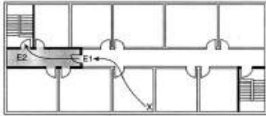
Contoh 3.18 - Jalan terusan eksit yang digunakan untuk menjaga jarak lintasan dari menjadi berlebihan. (sebagai penjelasan tambahan butir 3.9.2)
