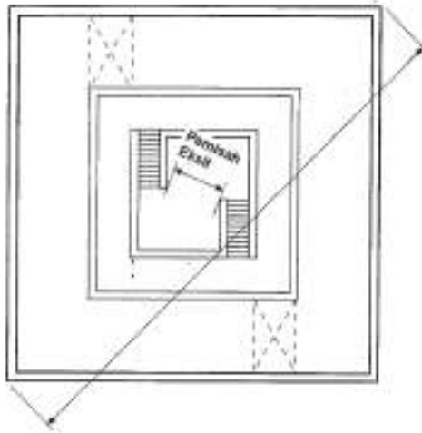
Gambar A.3.13.1.3.2.(c) - Pemisah eksit dan ukuran diagonal dari daerah yang dilayani.
