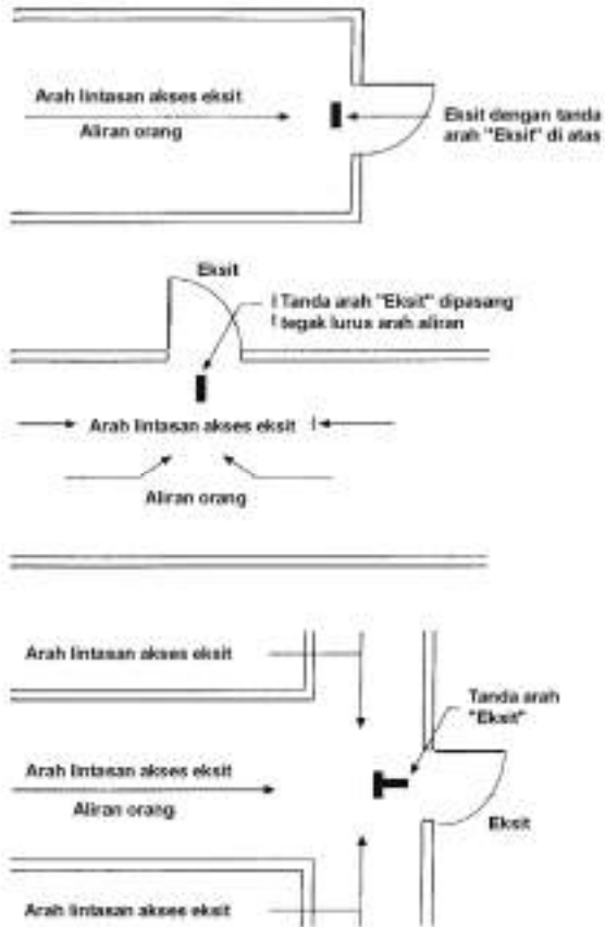
Gambar A.3.17.1.2 – Lokasi tanda arah Eksesit.
